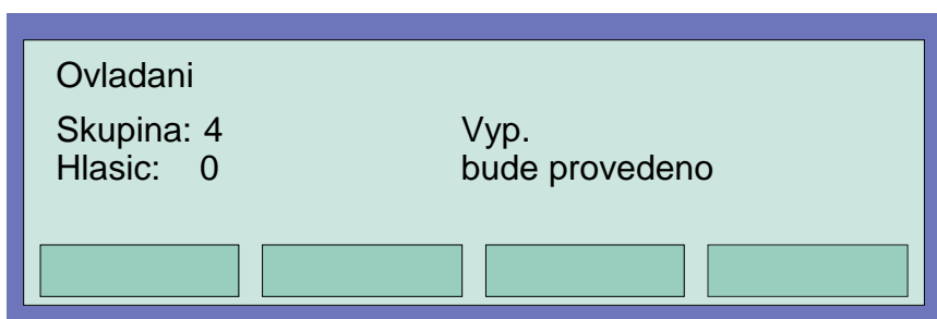
Obr. 17: Zobrazení na displeji při odpojení skupiny 4
