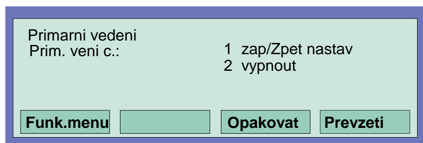
Obr. 44: Zadání čísla primárního vedení
