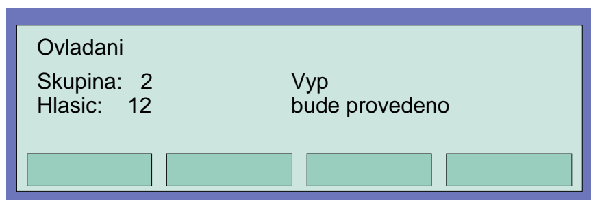
Obr. 24: Zobrazení na displeji při odpojení skupiny 2/hlásiče 12
