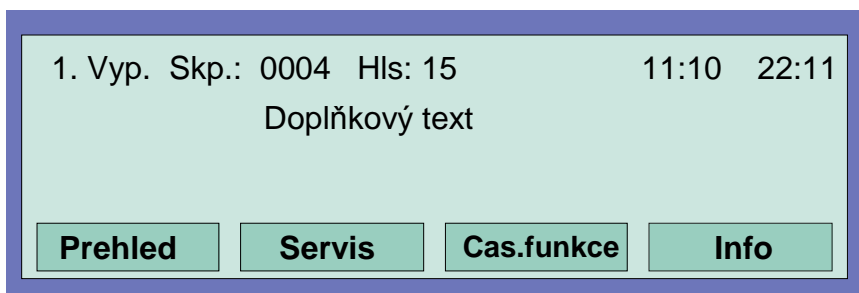
Obr. 18: Zobrazení na displeji ke hlášení odpojení v rámci stavového zobrazení
