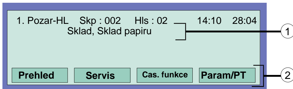
Obr. 34: Podrobné stavové zobrazení požáru (příklad)
