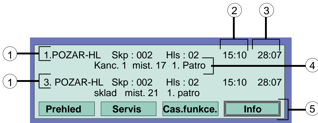
Obr. 10: Zobrazení hlášení požáru (příklad)
